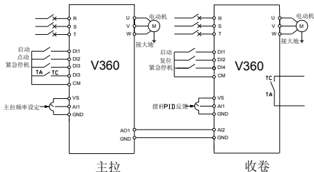
图 2-3 双变频拉丝机系统接线图
