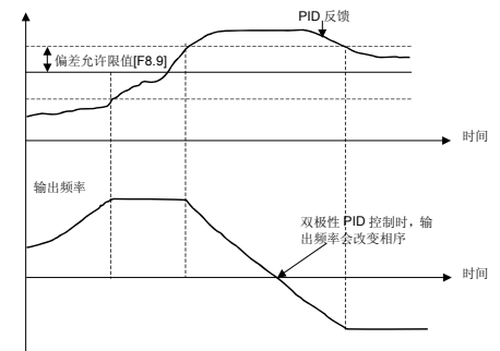
图 6-30 双极性 PID 控制方式
